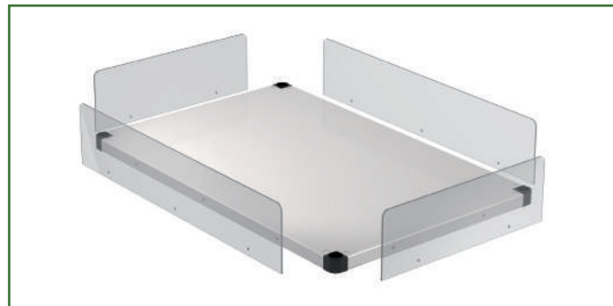
Kit sponde lexan su ripiano inferiore cavalletto Lexan sides kit for lower shelf of the stand Bandes en lexan sur l'étagère inférieure du chariot Lexan-Rändersatz zur unteren Ablage des Untergestells Kit bordes de lexan para el estante inferior del caballete
